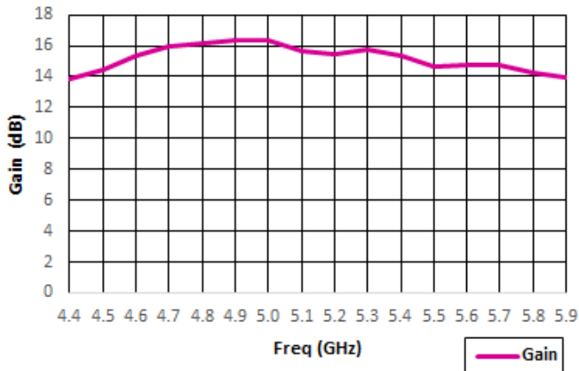
MGA-495940-02 Gain
